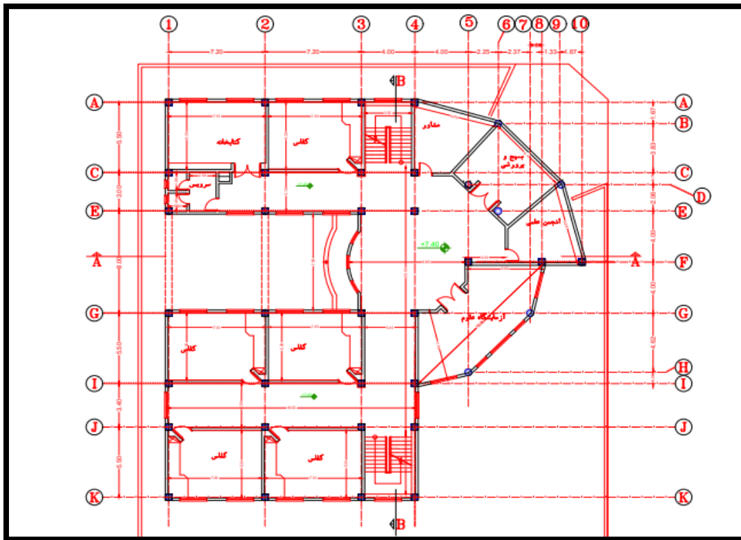
پلان طبقه اول
