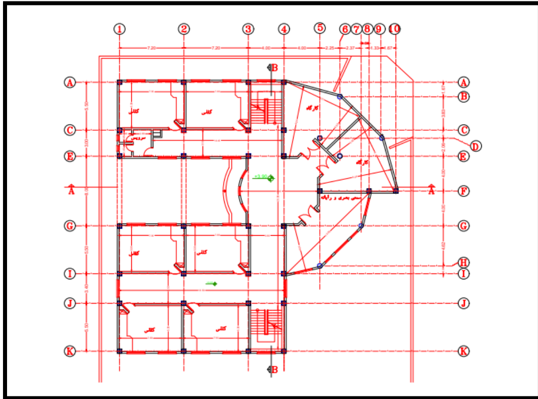
پلان طبقه اول
